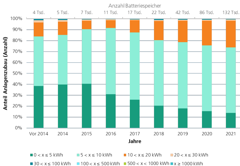
Batteriespeicher – Anlagenzubau (zahlenmäßig) nach Kapazitätskategorien. © Fraunhofer ISE
